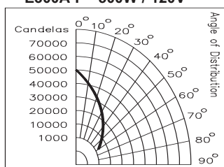
E300A-F - 500W / 120V
